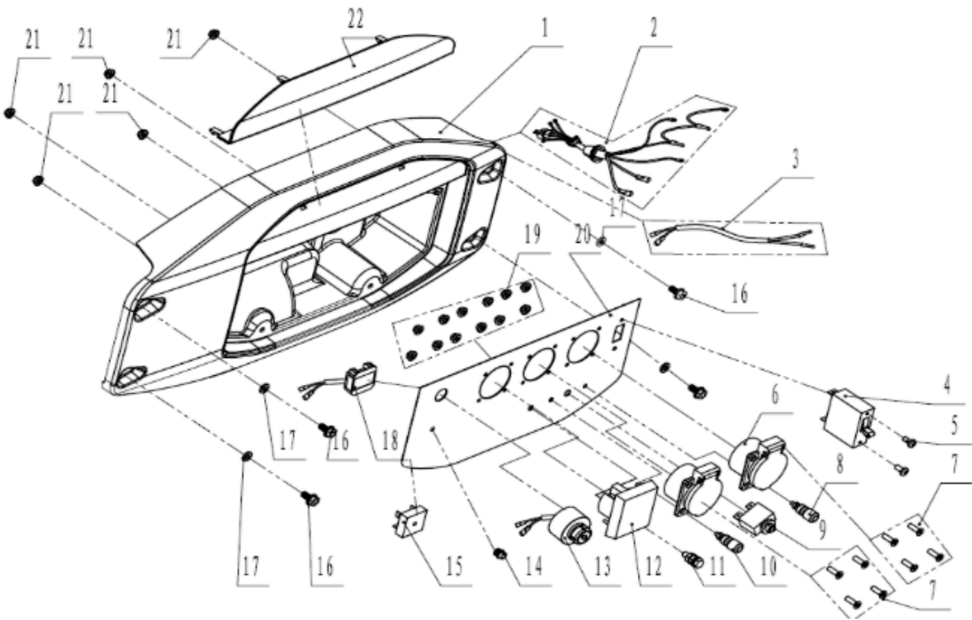
面板组件（电启动） Panel component (electric start)
