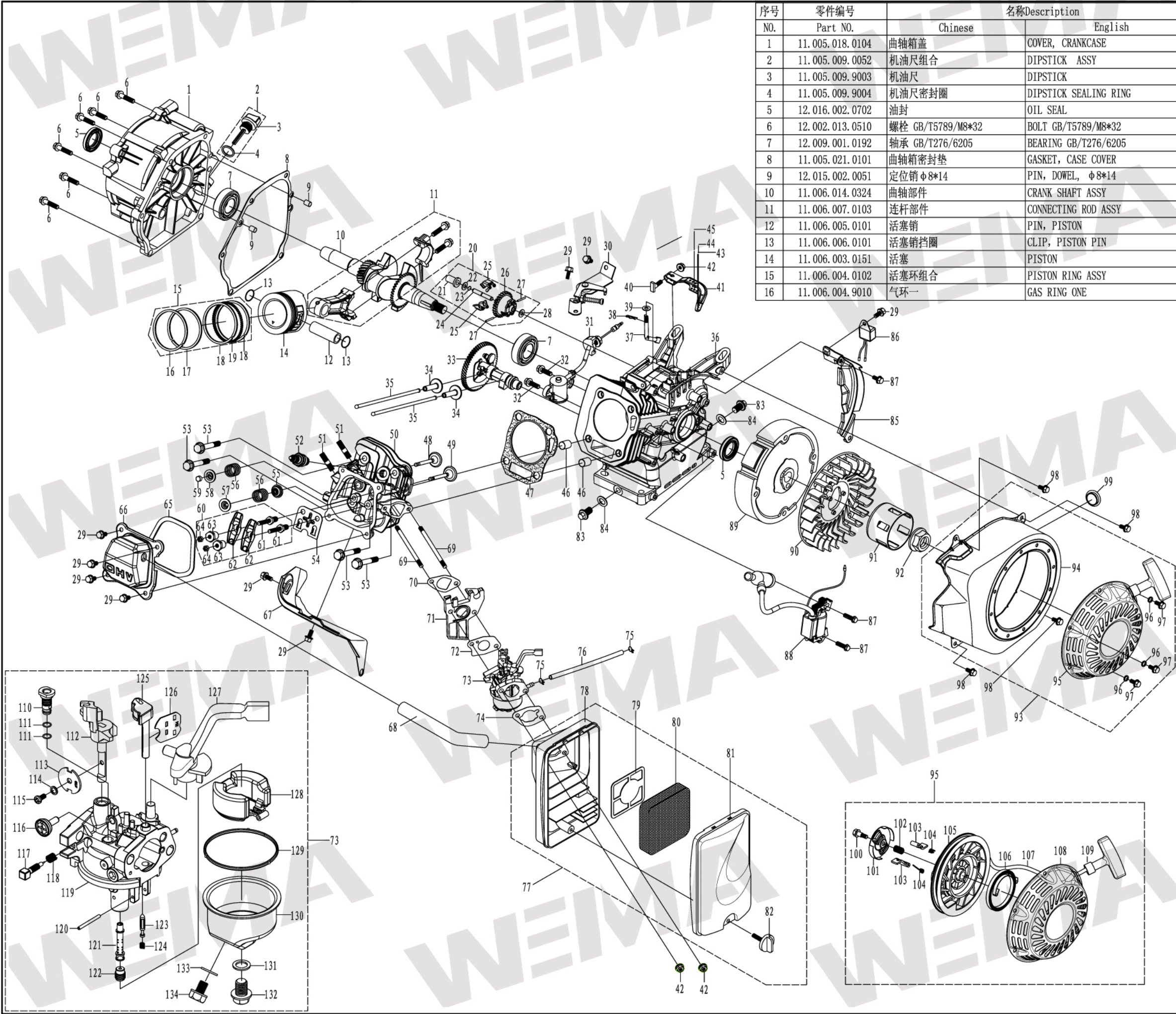
WM168FB/P机组动力爆炸图
